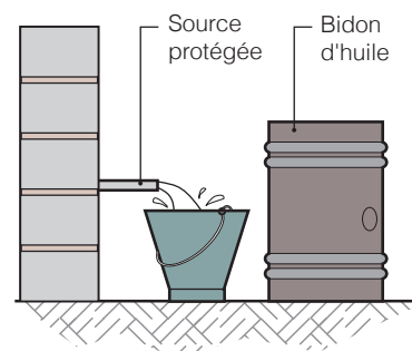
Figure 34. Le type de récipients utilisé par les communautés doit être intégré dans la conception du point d'eau
