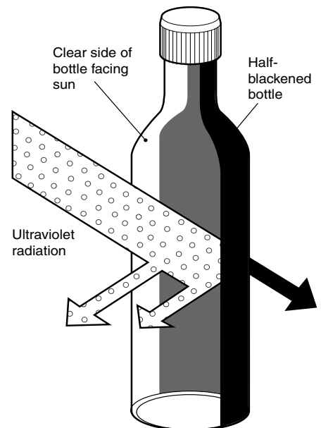
The SODIS system
